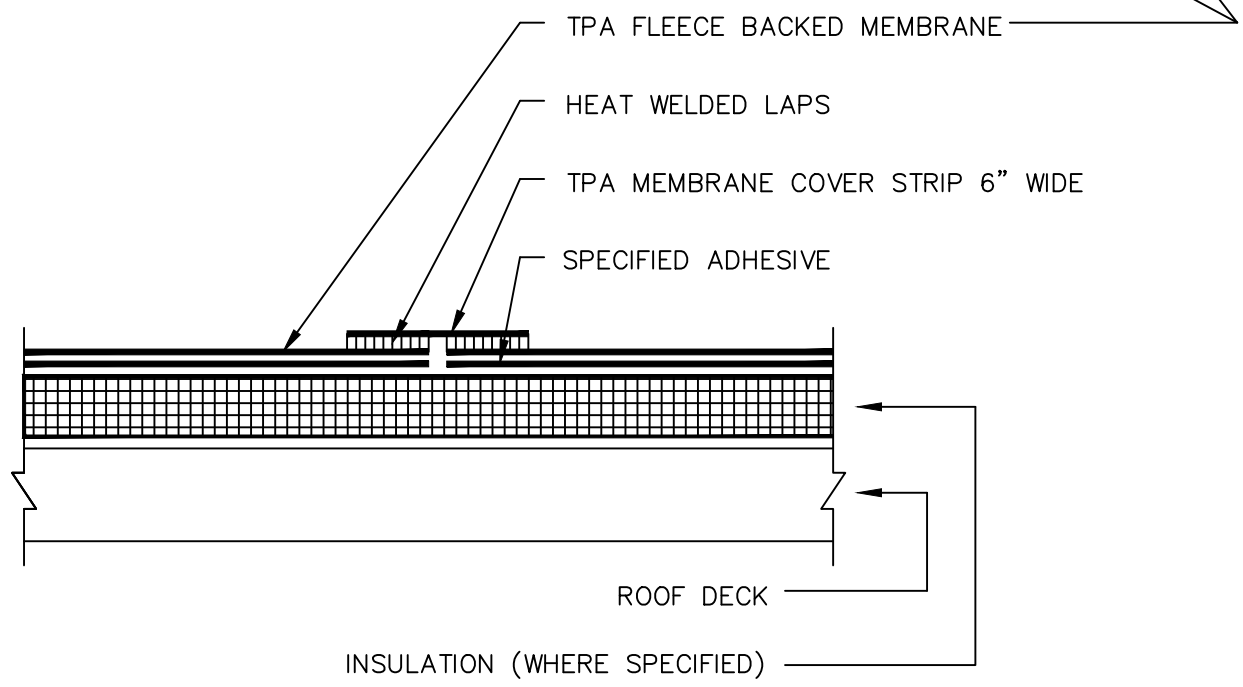
SECTION A-A
